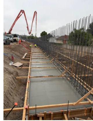
Los equipos vierten hormigón para construir la base del nuevo muro acústico.
