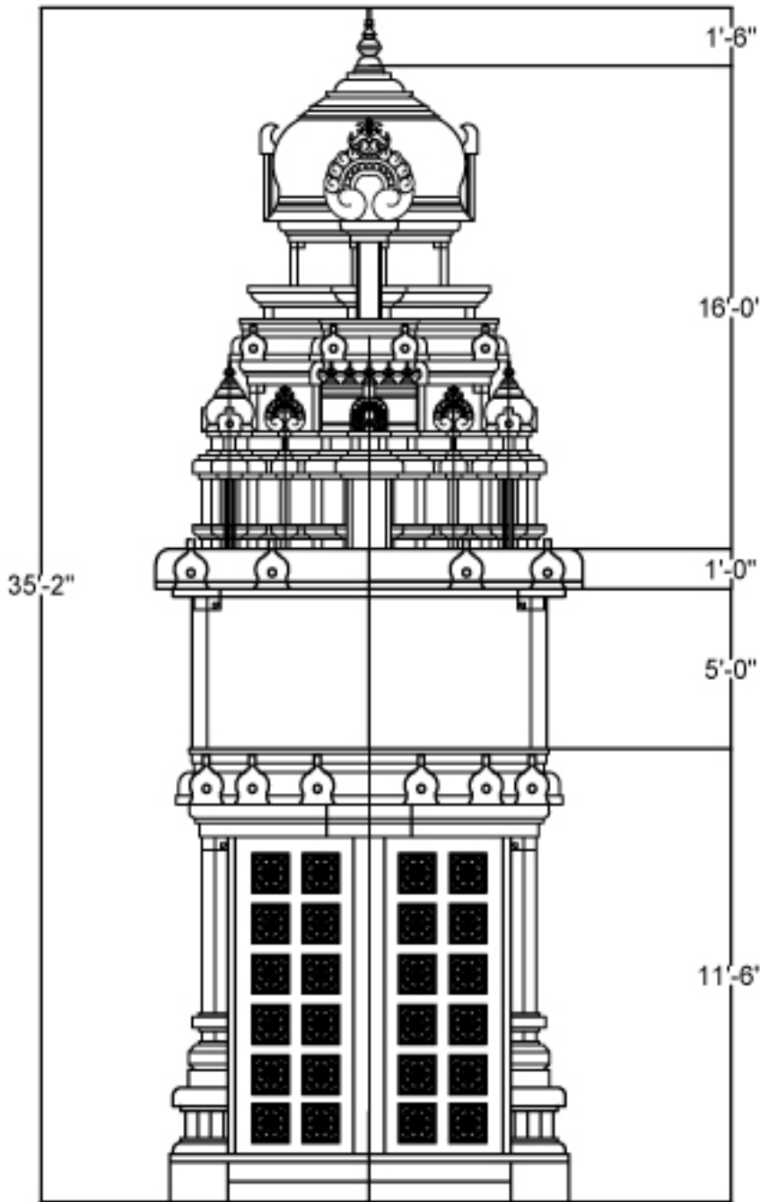
ELEVATION
