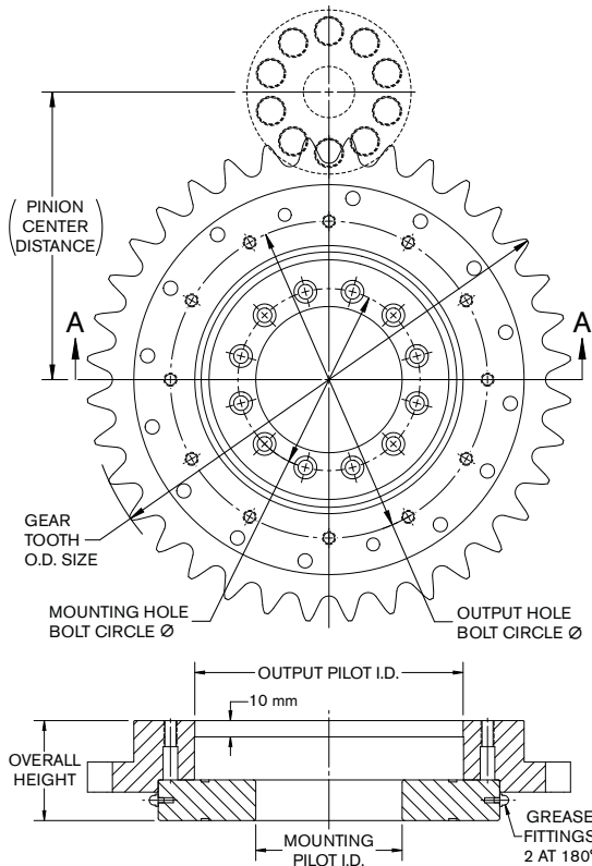
SECTION A-A
